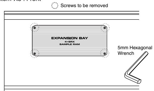
Fantom-X8 : Front
