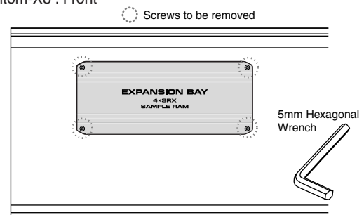
Fantom-X8 : Front
